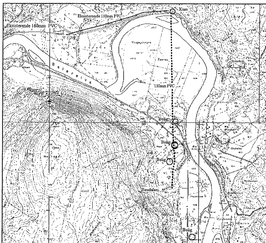
Figur 1. Prinsippskisse ved fremføring av kommunalt vann fra Larsos til Nes. Boliger med rund sirkel.
